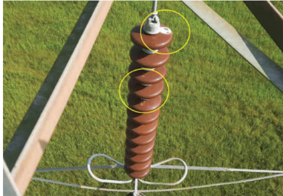
ကေဗွီ ၂၃၀ ကမာနုတ်-စစ်တောင်း ဓာတ်အားလိုင်းထိန်းသိမ်း ပြုပြင်ခြင်းလုပ်ငန်းဆောင်ရွက်ရမည့် မှတ်တမ်းဓာတ်ပုံ။
